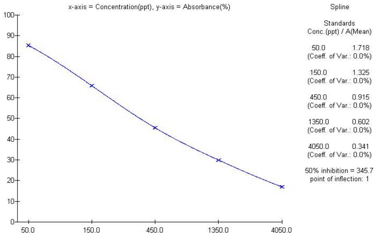
标准曲线图
